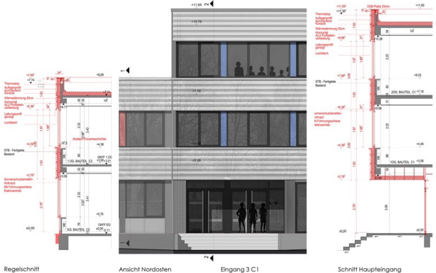
Detailansicht, Schnitt
