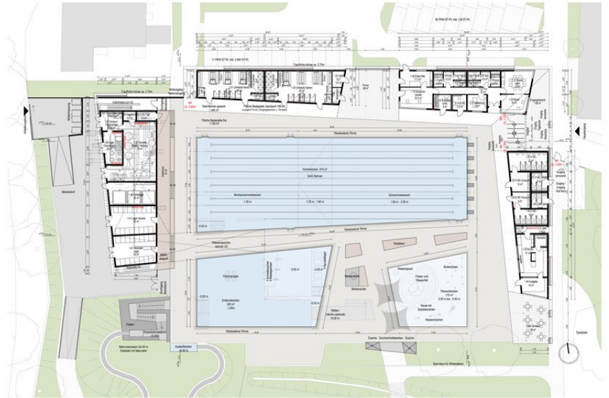
Grundriss EG
