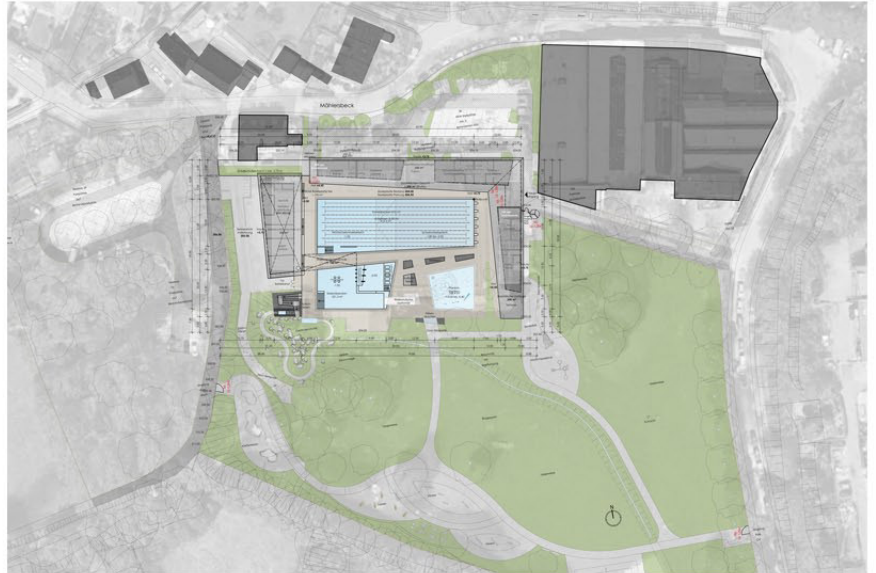
Lageplan
